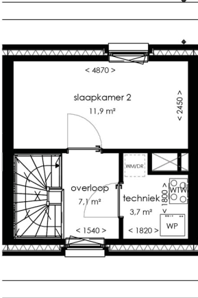
tweede verdieping
