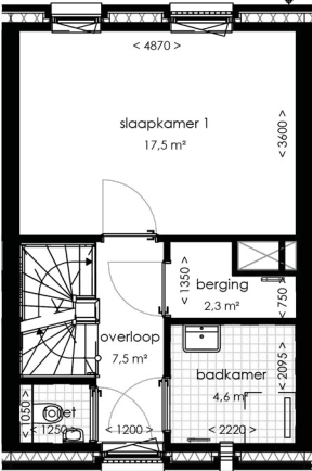
eerste verdieping
