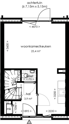
beginne grond
