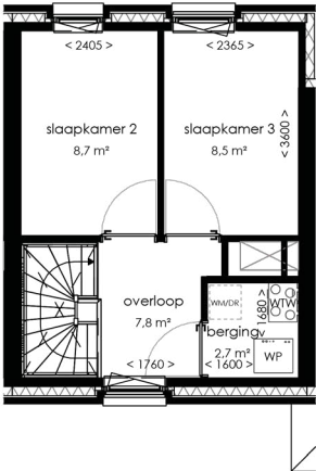
tweede verdieping
