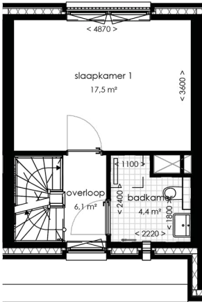
eerste verdieping
